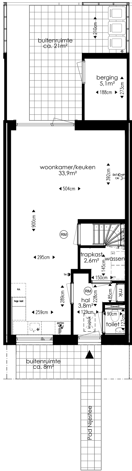
Begane grond
